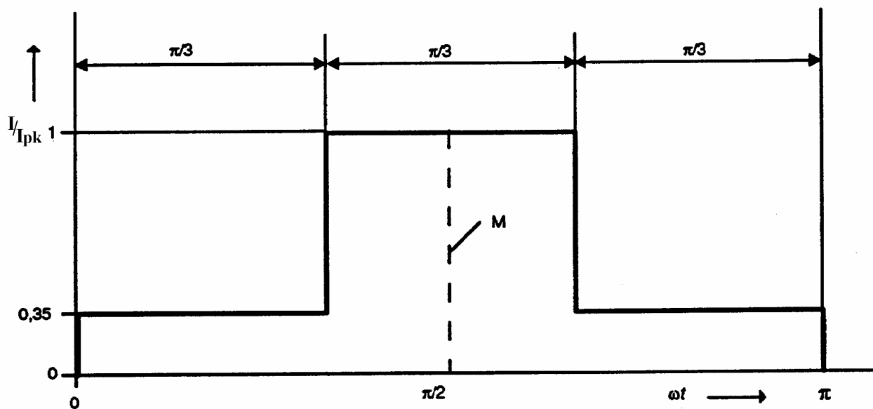
Рисунок 1 – График для определения «специальной формы кривой» потребляемого тока и отнесения ТС к классу D
